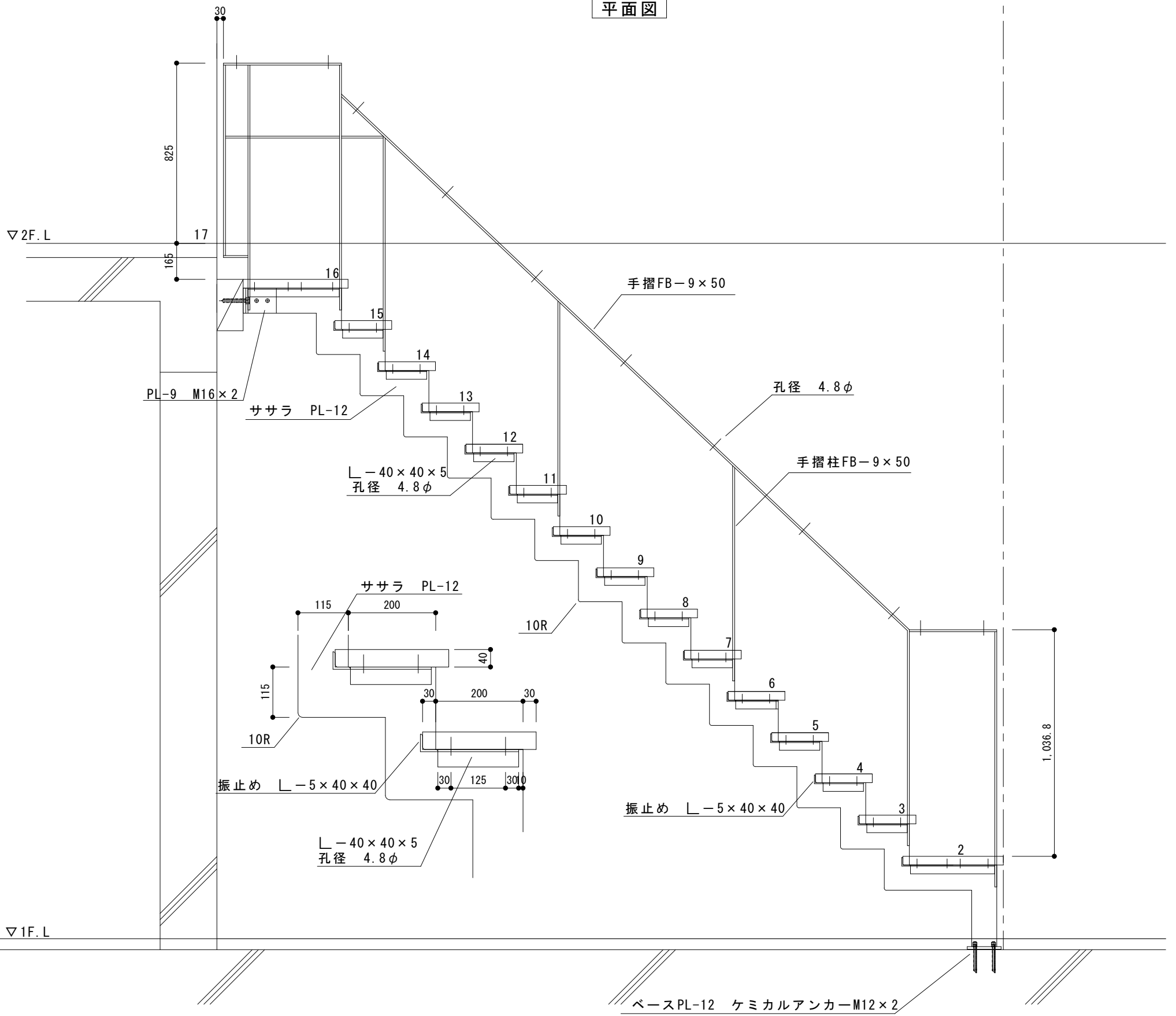
立面図
