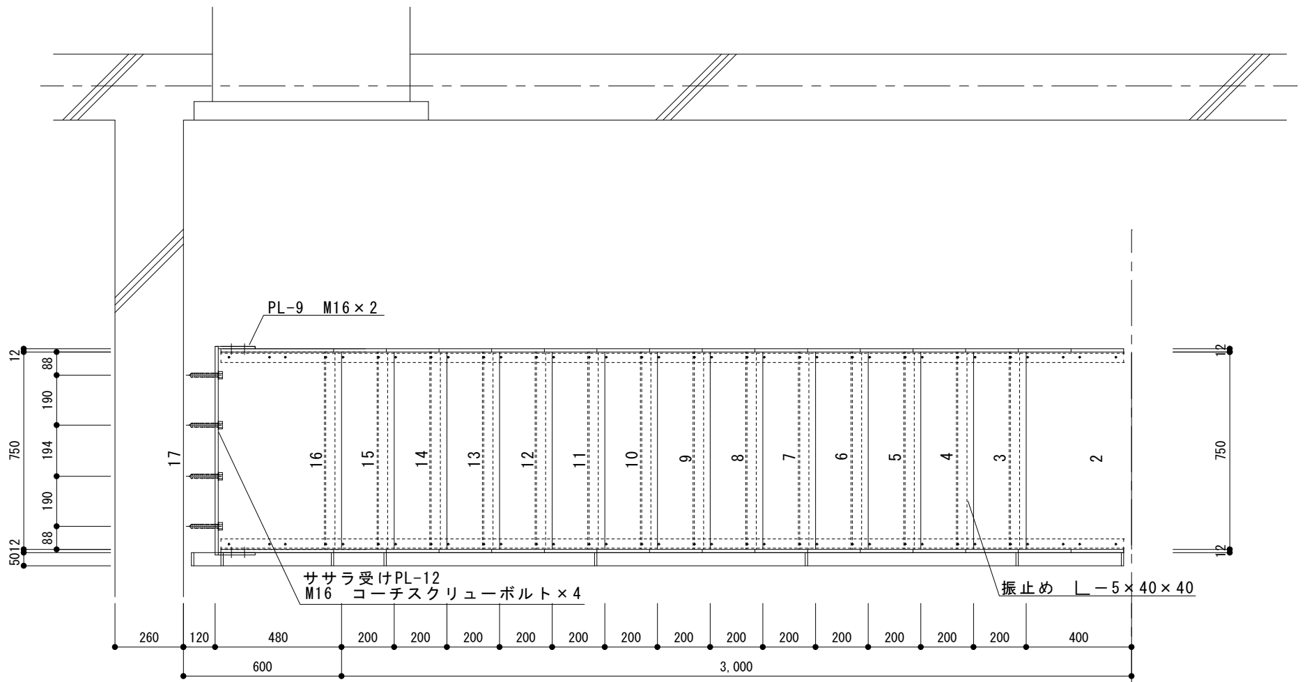
平面図
